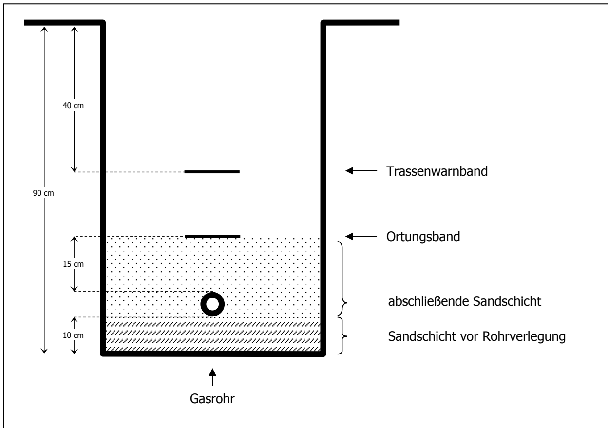
Abbildung: Schnittdarstellung - Rohrgraben
